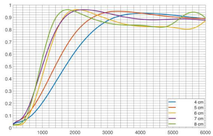
Simulatie van de geluidsabsorptiecoëfficiënt met Thomasson-correctie
