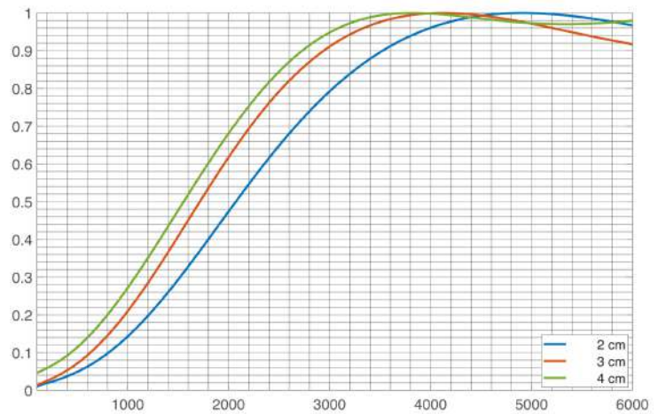
Simulatie van de geluidsabsorptiecoëfficiënt met Thomasson-correctie
